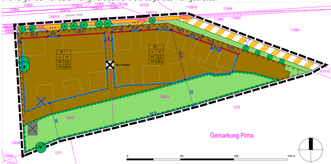
Abb.: Planzeichnung Bebauungsplan Nr. 92 „An der Dresdner Straße“ der Stadt Pirna
