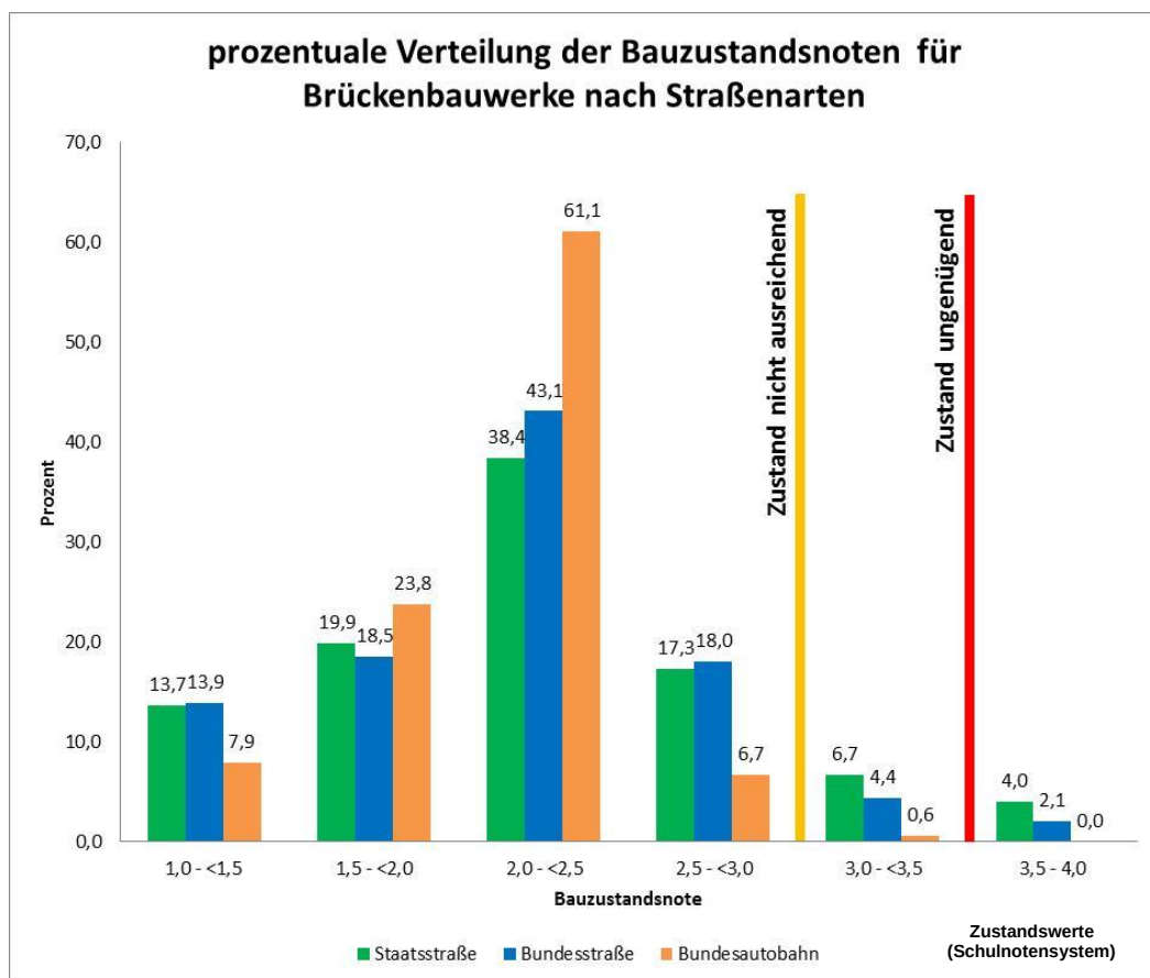
Abbildung 4: Zustand der Brücken im Freistaat Sachsen 4
