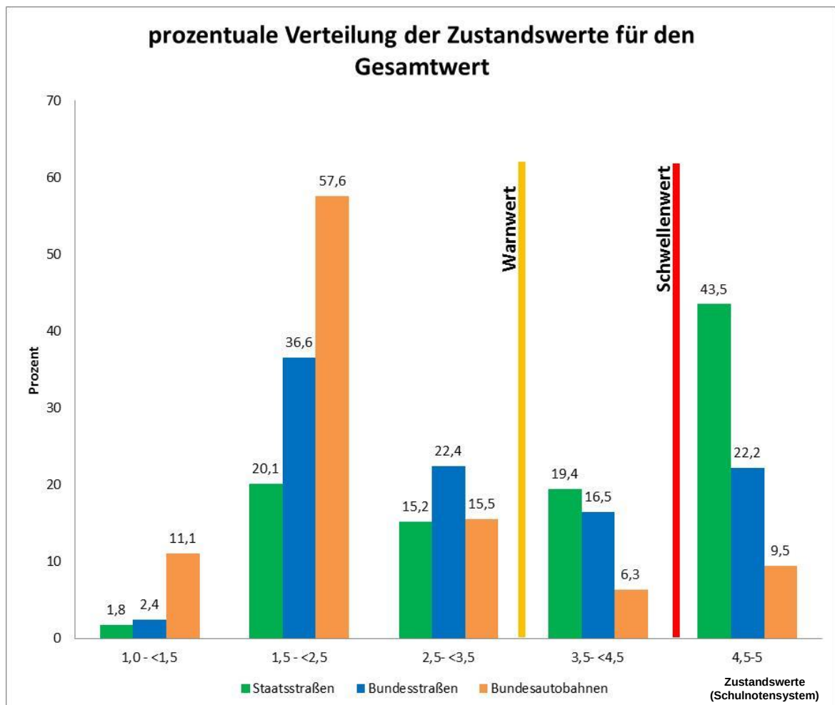
Abbildung 3: Zustand der Staats-, Bundesstraßen und Bundesautobahnen im Freistaat Sachsen
