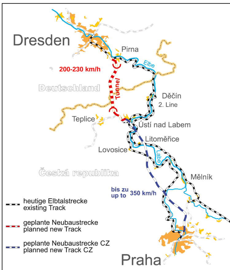
Abbildung 17: Neubaustrecke Dresden - Prag
