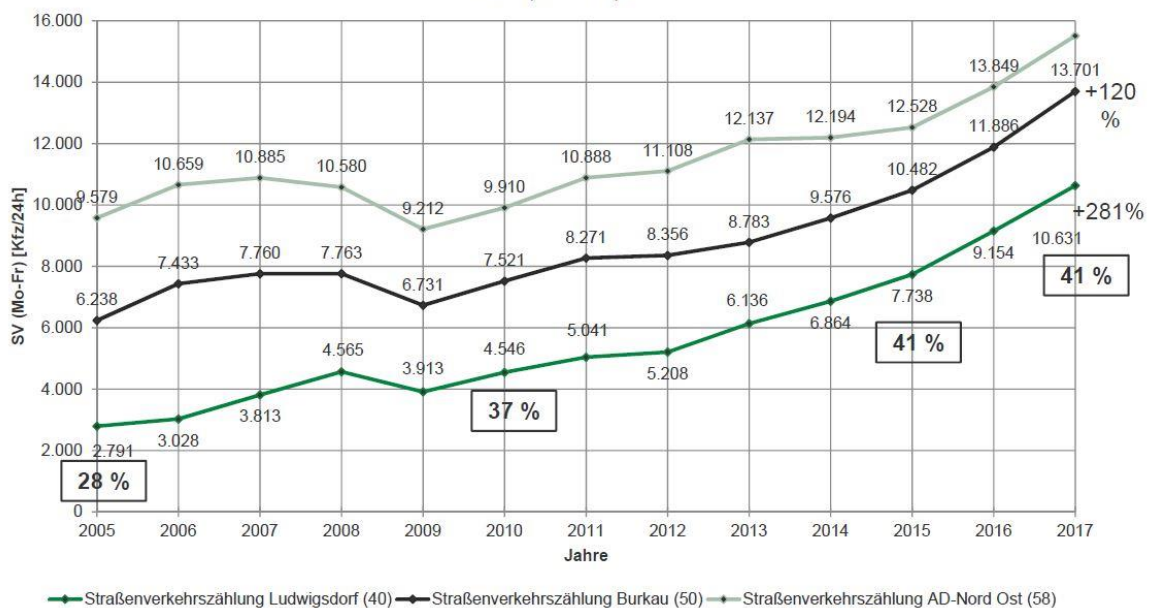
Abbildung 8: Entwicklung Verkehrsaufkommen (DTV) und Schwerverkehrsanteil (SV) – BAB A4 (AD Dresden-Nord bis Landesgrenze D/PL), Zählstellen Ludwigsdorf, Burkau, AD Nord-Ost
